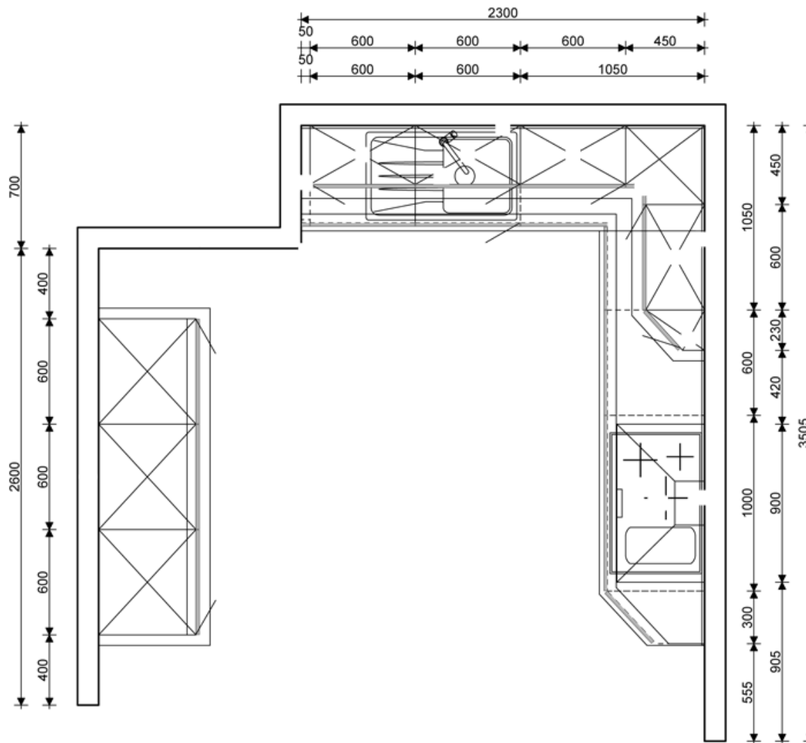
Musterküche KD-24
