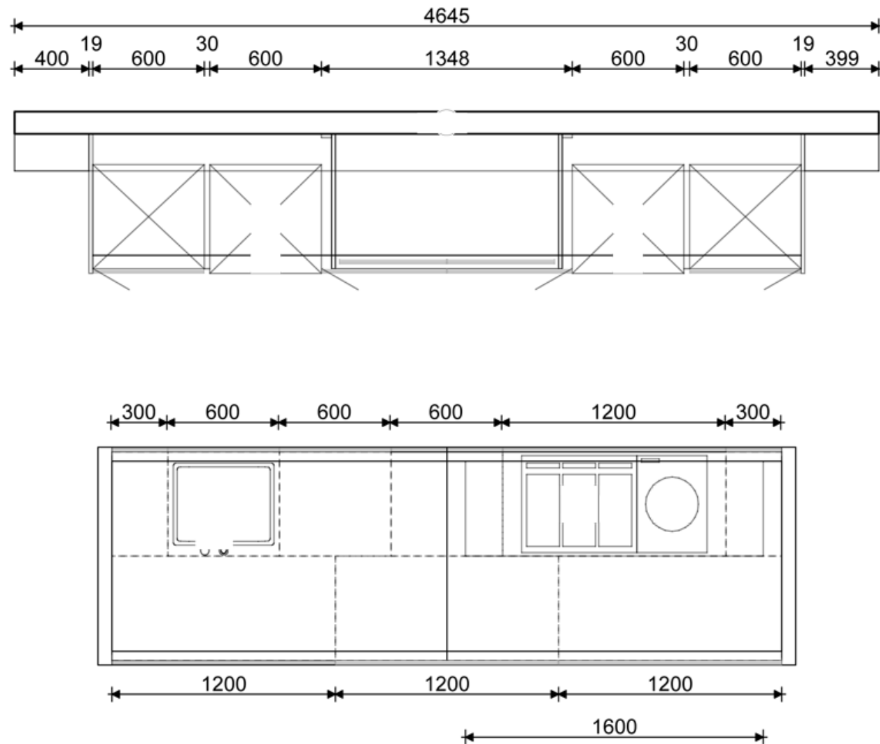
Musterküche BI-58
